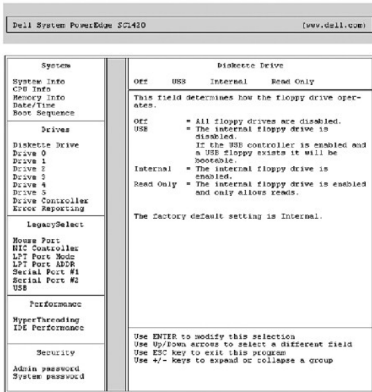
그림 3-1. 시스템 설치 프로그램 기본 화면
