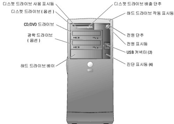
그림 1-1. 전면 패널 구조 및 표시등
