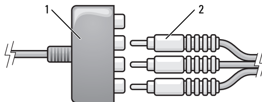
1 元件影像配接器 2 元件影像纜線
