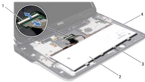
1 鍵盤纜線連接器 2 鍵盤 3 鍵盤彈片 (4) 4 頂蓋
