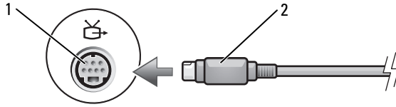
1 S-Video-TV-Ausgang 2 S-Video-Anschluss
