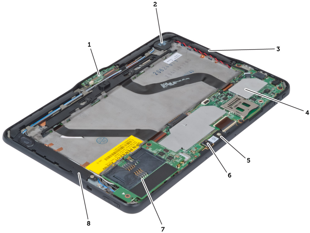
그림 2. 내부 보기
