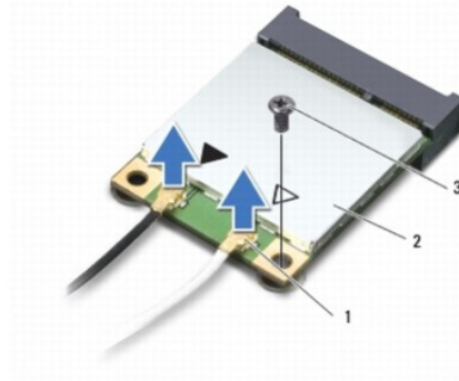
1 מחברים לכבל אנטנה (2) Mini-Card 3 בורג
