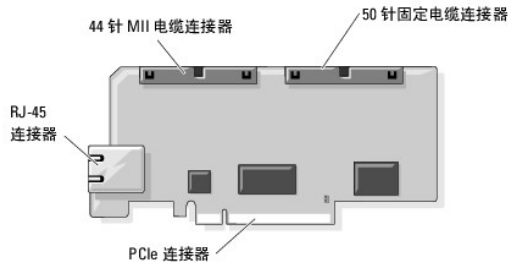
图 1-1. DRAC 5 硬件功能
