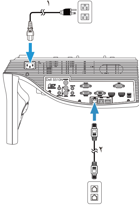
شبكة الاتصال المحلية (LAN)
