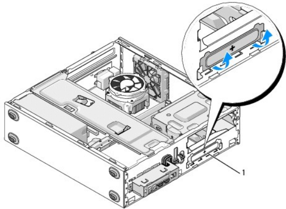
1 แผ่นโลหะชนิดทึบทั้งของช่องขนาด 3.5 นิ้ว
