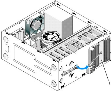
1 แผ่นโลหะของช่องขนาด 5.25 นิ้ว (สำหรับช่องไดรฟ์ออปติคัลที่ว่างเปล่า)
