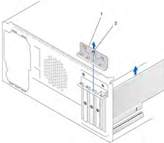
1 זוויתן לקיבוע הכרטיס 2 בורג
