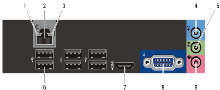
图 3: 小型塔式机和台式机的背面板视图
